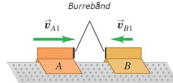
(a) Før kollision
